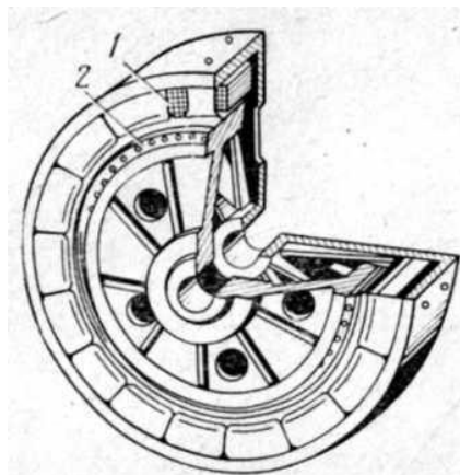
Рис. 3. Общий вид электромагнитной муфты скольжения.
