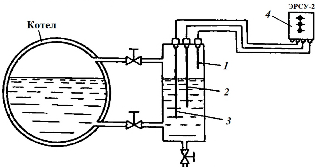
Рис. 3. Электродный сигнализатор уровня типа ЭРСУ-2
