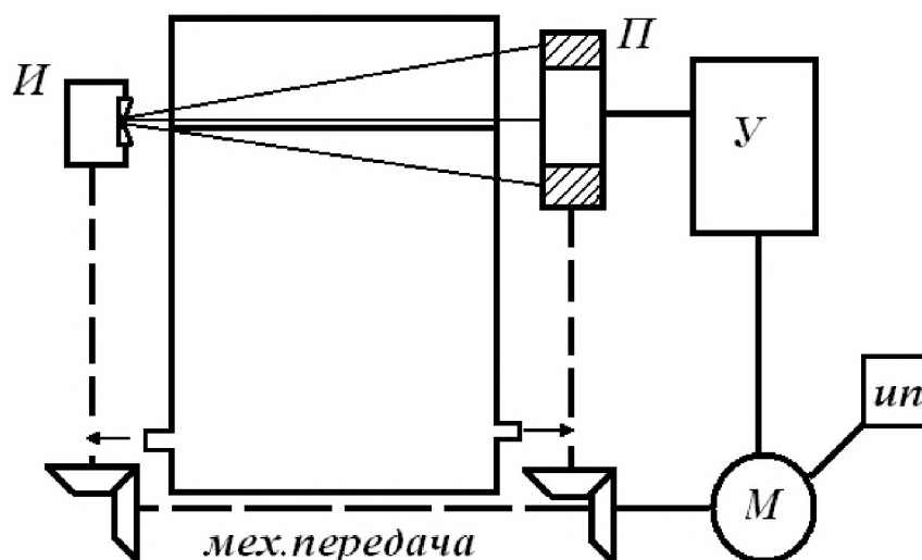
Рис. 5. Принципиальная схема радиоизотопного уравнимера
