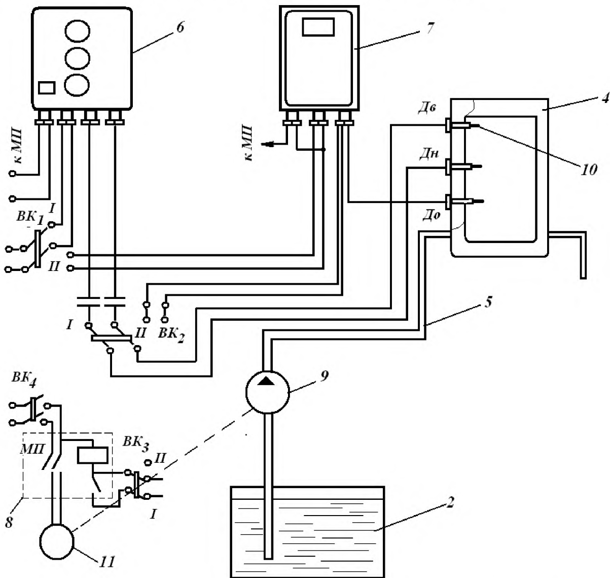
Рис. 7. Принципиальная электрическая схема лабораторной установки
