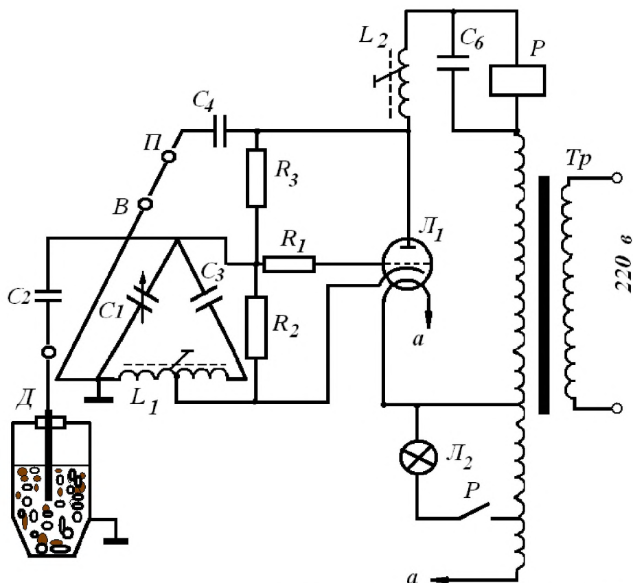
Рис. 4. Принципиальная схема электронного сигнализатора уровня ЭСУ-1М
