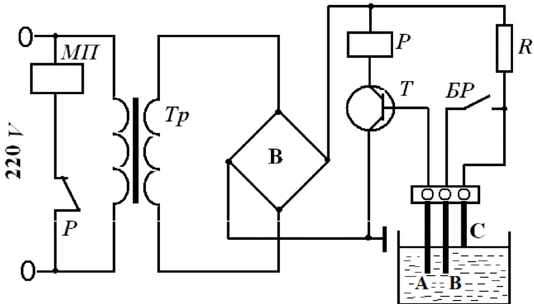
Рис. 2. Регулятор уровня с электродными датчиками
