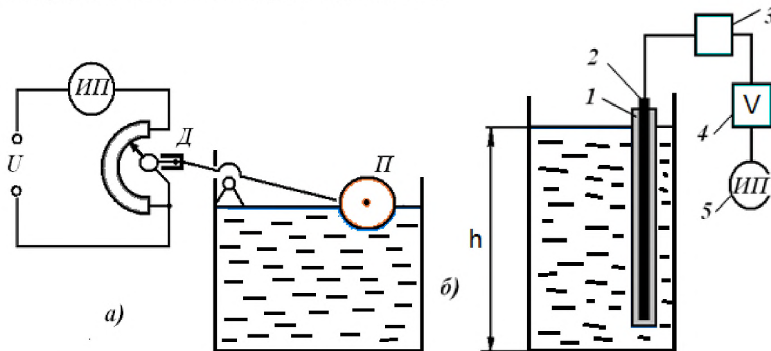
Рис. 1. Схемы уровнемеров:
