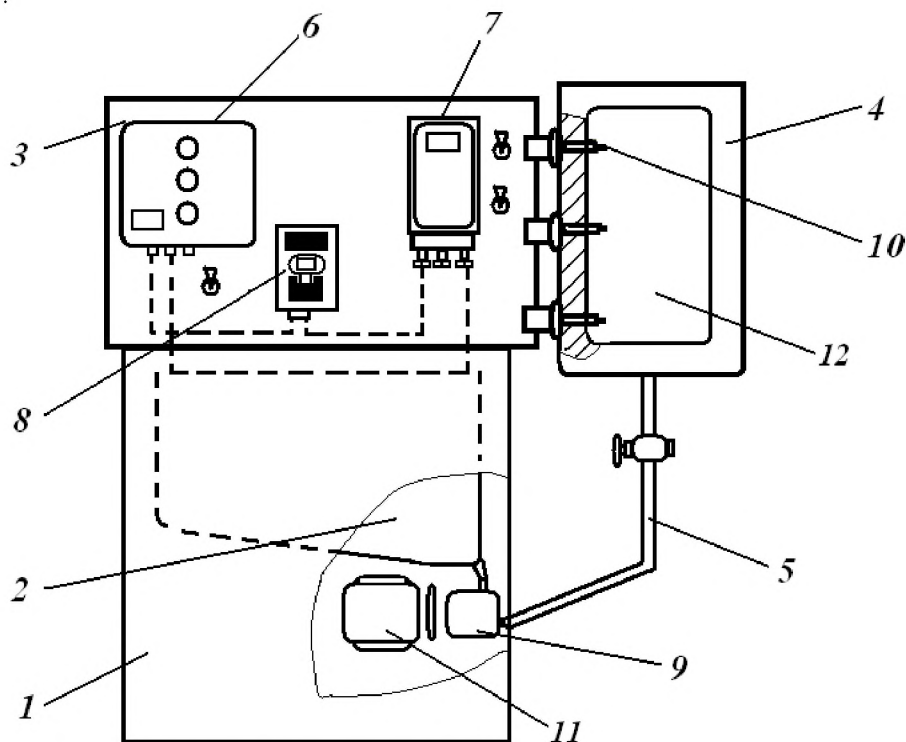
Рис. 6. Общий вид лабораторной установки
