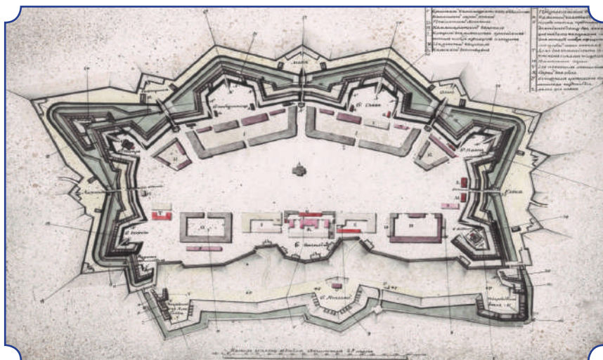
Рисунок 5. План Тираспольской Срединной крепости
