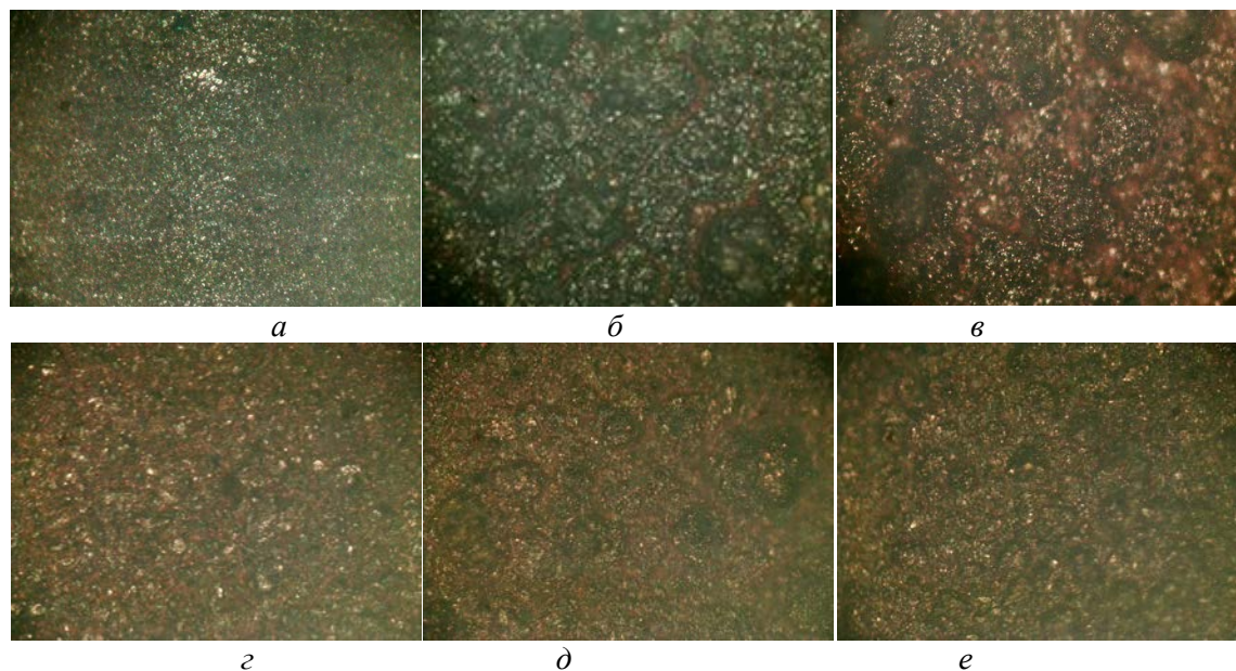
Рис. 7. Микрофотографии морфологии медных покрытий (250-х): а – электролит № 1 плотность тока 1 А/Дм 2 ; б – электролит № 1 плотность тока 6 А/Дм 2 ; в – электролит № 1 плотность тока 7 А/Дм 2 ; г – электролит № 2 плотность тока 1 А/Дм 2 ; д – электролит № 2 плотность тока 6 А/Дм 2 ; е – электролит № 2 плотность тока 7 А/Дм 2
