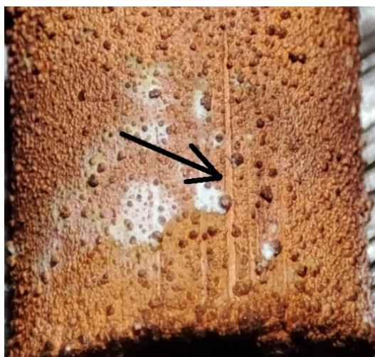
Рис. 10. Цилиндрический образец без изоляции кромок (5 А/Дм 2 , электролит № 1)
