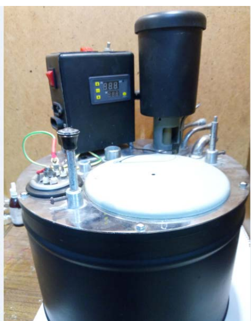
Рис. 1. Электролитическая ячейка
