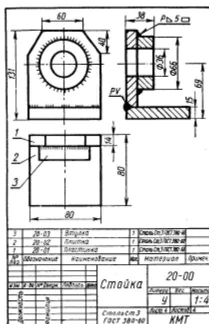
Примеры выполнения чертежей сварных соединений
