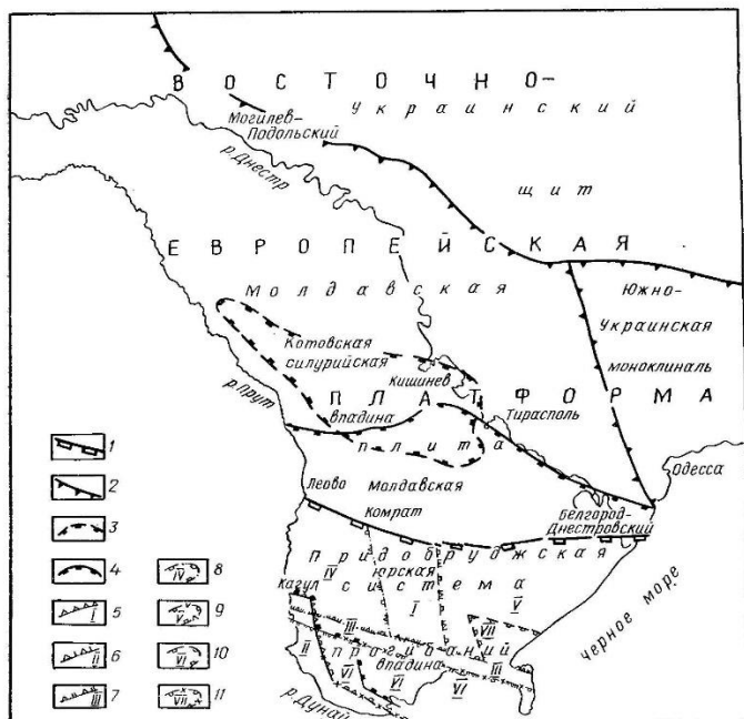
Рисунок 1. Схема тектонического районирования Днестровско-Прутского междуречья
