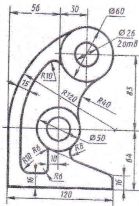
Станина
