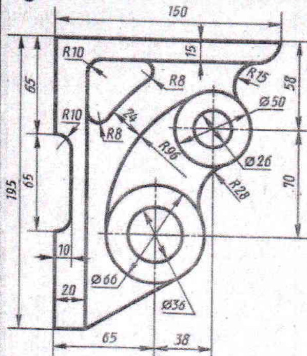
Кронштейн
