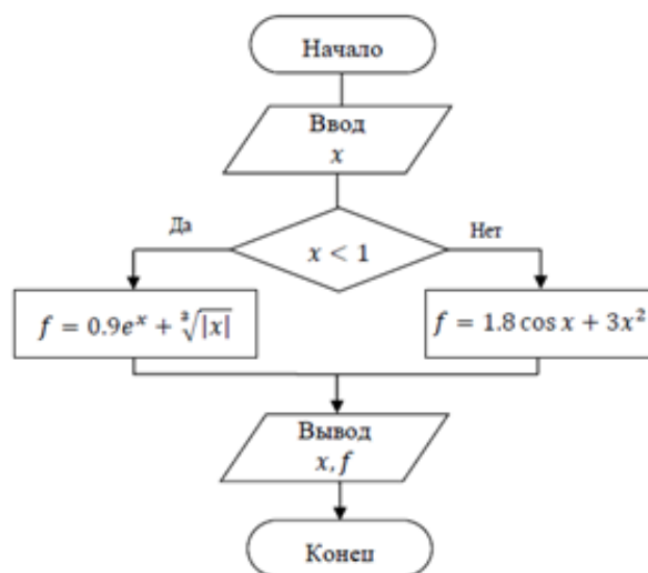
Блок-схема алгоритма
