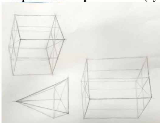
Комбинаторика
