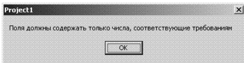
Рис. 2.6. Пример ошибки
