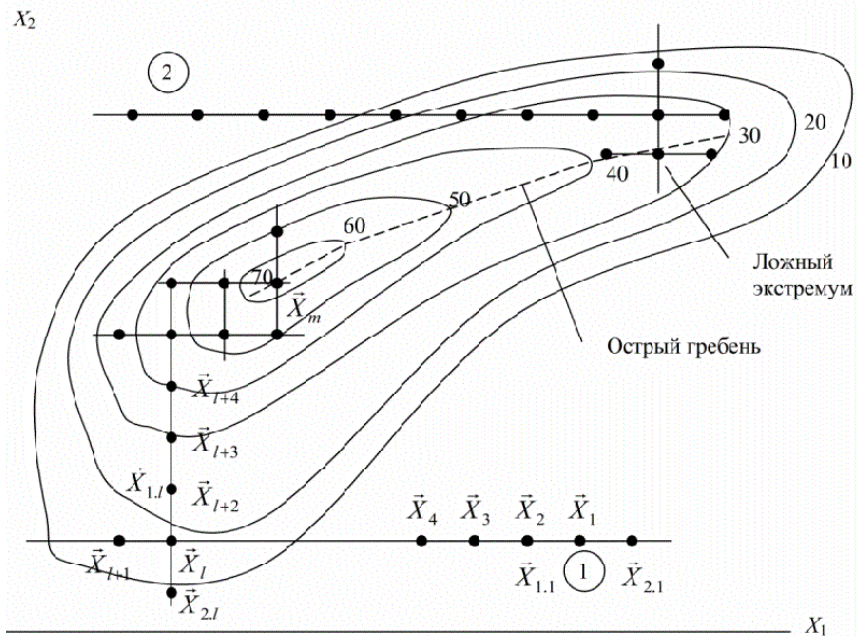
Рис. 1.1. Ход процесса поиска экстремума
