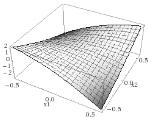
Рис. 2.8. Гиперболический параболоид
