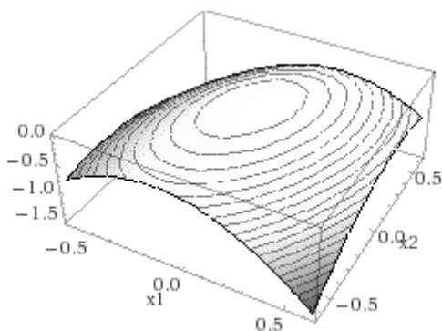
Рис. 2.7. Эллиптический параболоид
