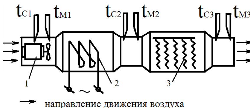
Рис. 2. Схема установки для изучения свойств влажного воздуха 1 – вентилятор с двигателем, 2 – электроподогреватель, 3 – сушильная камера; t_C и t_M – соответственно показания сухого и мокрого термометров
