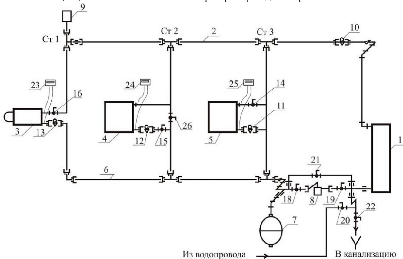
Рис. 1. Схема лабораторной установки
