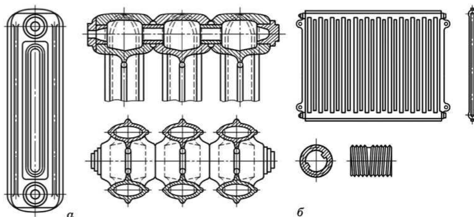
Рис. 8. Отопительные радиаторы: а) чугунные; б) стальные штампованные
