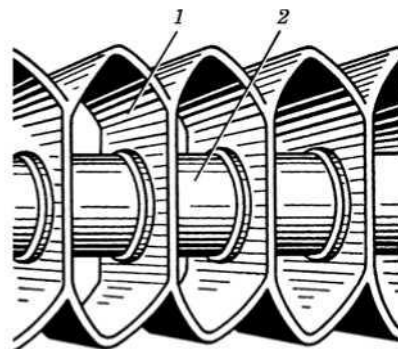
Рис. 10. Конвекторы плитного типа: 1 — ребристый элемент; 2 — труба
